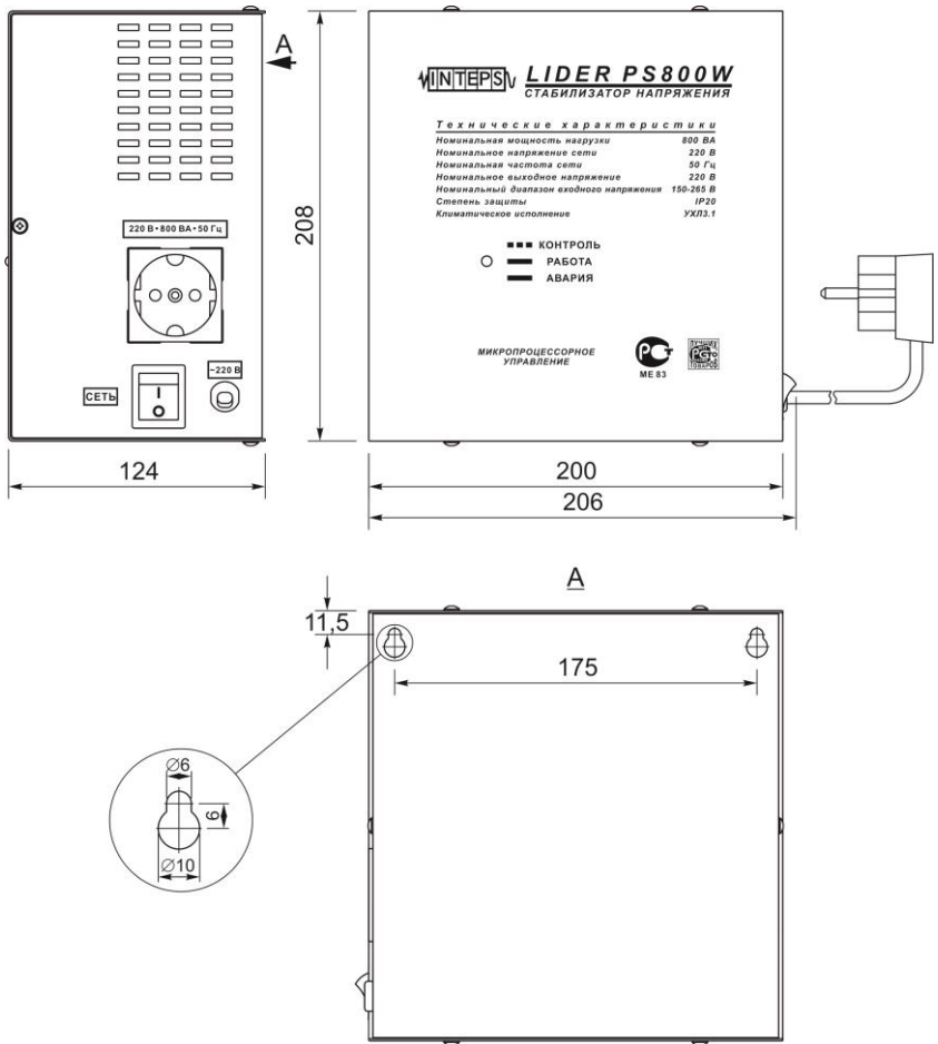
Габаритные и установочные размеры стабилизаторов напряжения переменного тока LIDER PS800W
